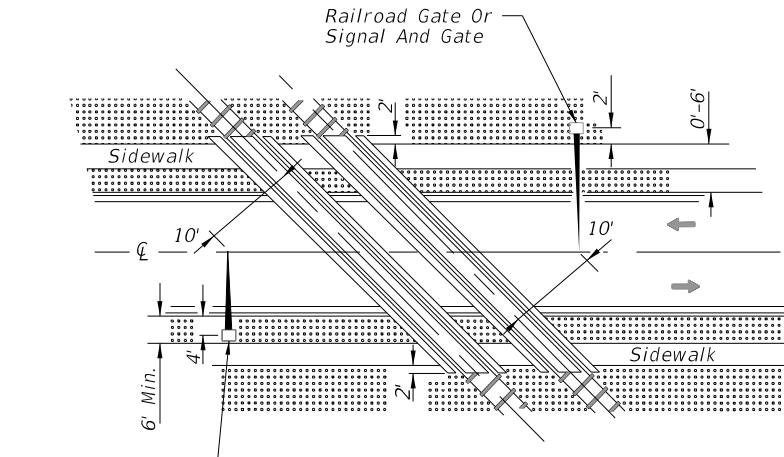
OBTUSE ANGLE
